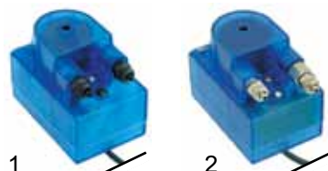
Technická data: Typ: Mybo Připojení hadice: 4x6mm
