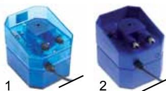
Technická data: Typ: Protho Druh ochrany: IP55 Připojení hadice: 4x6mm Míry: B-11 T-109 H-130
