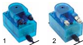
Technická data: Typ: Mybo Druh ochrany: IP65 Připojení hadice: 4x6mm
